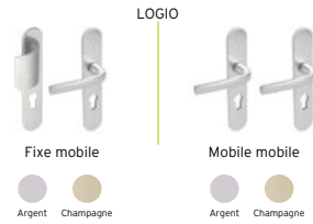
Fixe mobile entraxe 195 mm
